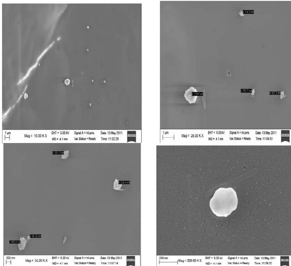
Fig. 2 (a), (b), (c) and (d) FESEM of PMMA/Al 2 O 3
