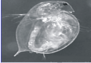
Fig. 1a: Ceriodaphnia
