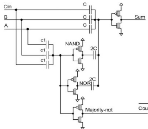
Fig.3 CNFET FA2
