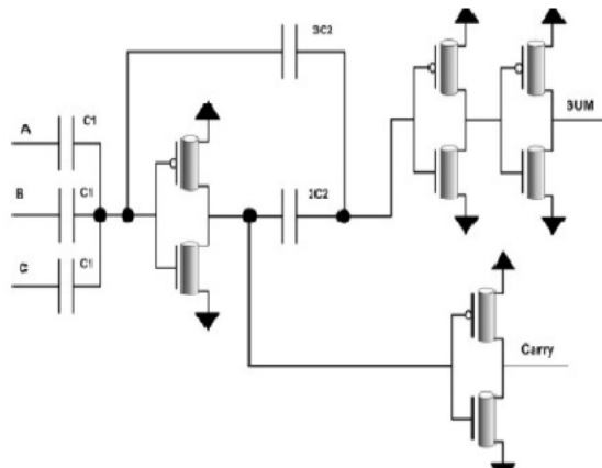
Fig.3 CNFET FA2
