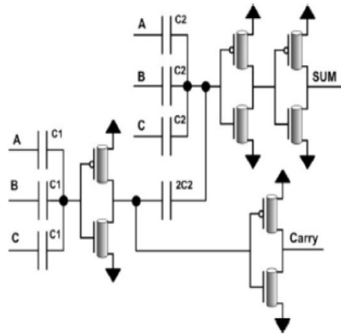
Fig.2 CNFET FA1
