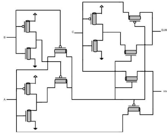
Fig.5 CNFET FA-4
