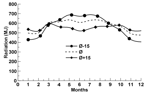
Fig 8. Monthly average solar radiation for latitude angle and latitude angle±15
