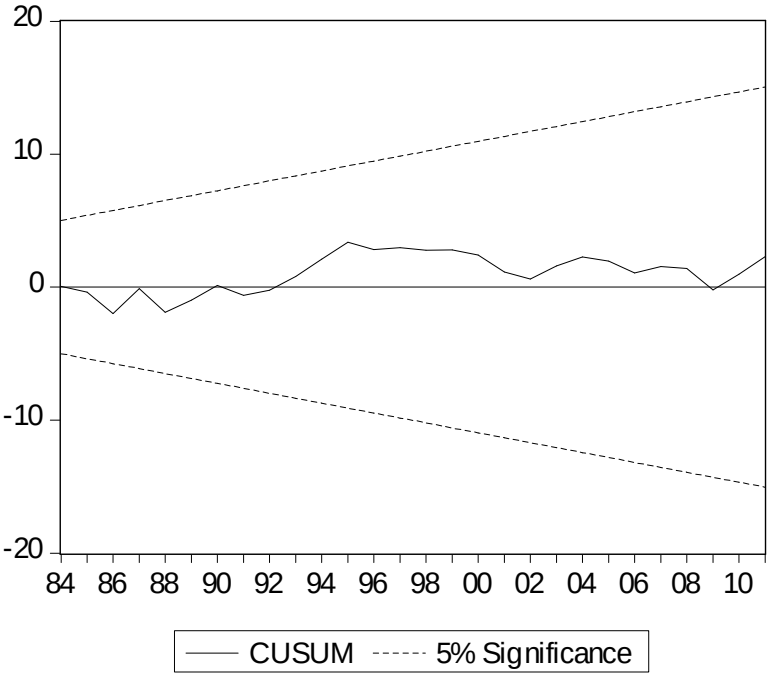
391 392 393 Fig. 3. Stability test for parameter 394 395 .
