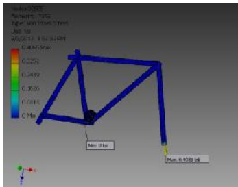
Figure: Von mises Stress
