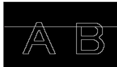
287 288 289 290 291 292 293 294 295 296 297 298 299 300 301 Fig. 11. Initial straight solution path for 'AB'
